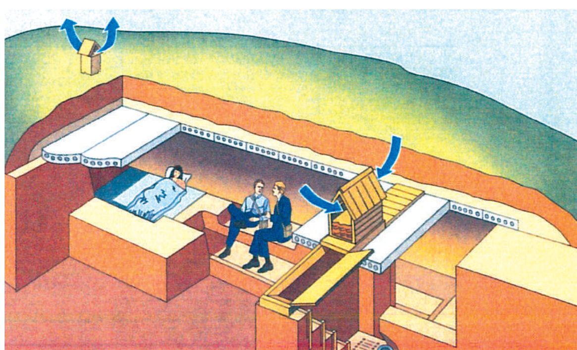
Быстровозводимое противорадиационное укрытие из железобетонных плит
